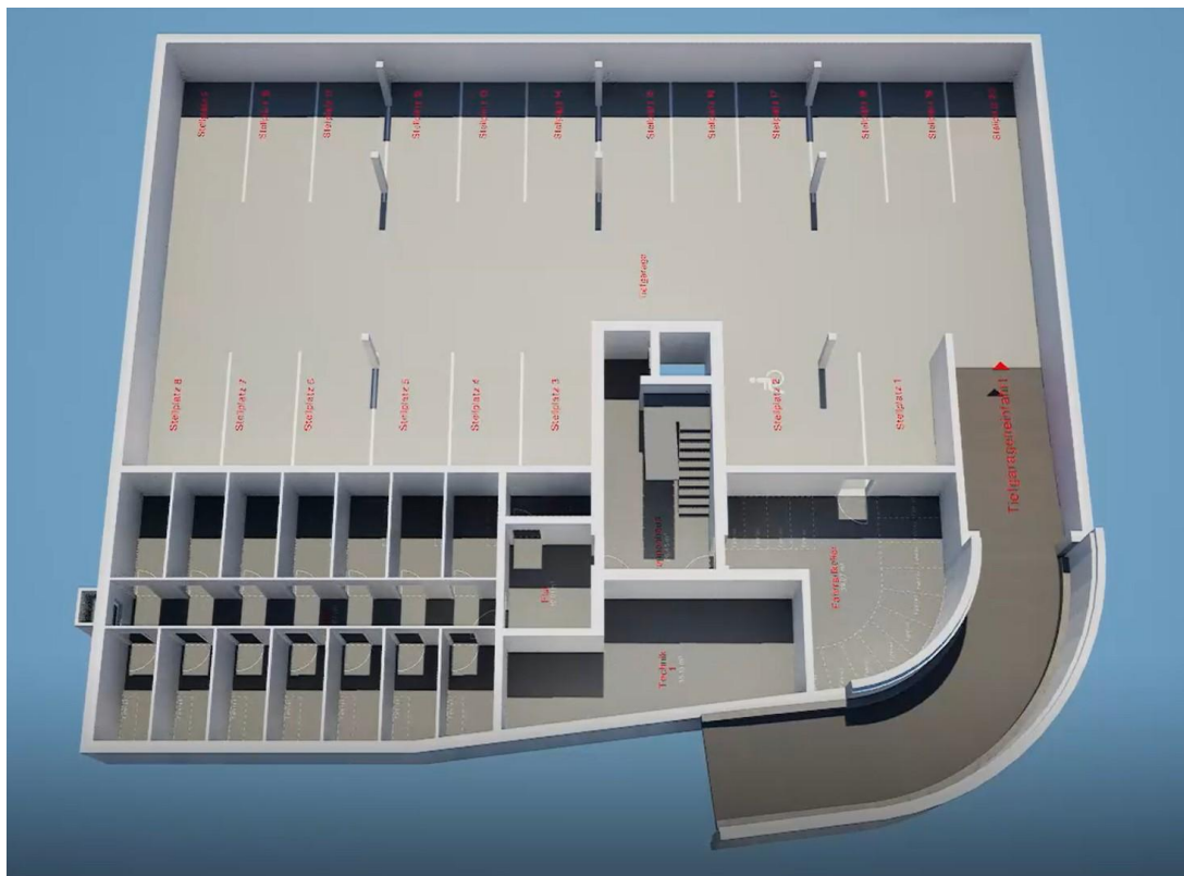
Grundriss Untergeschoss
