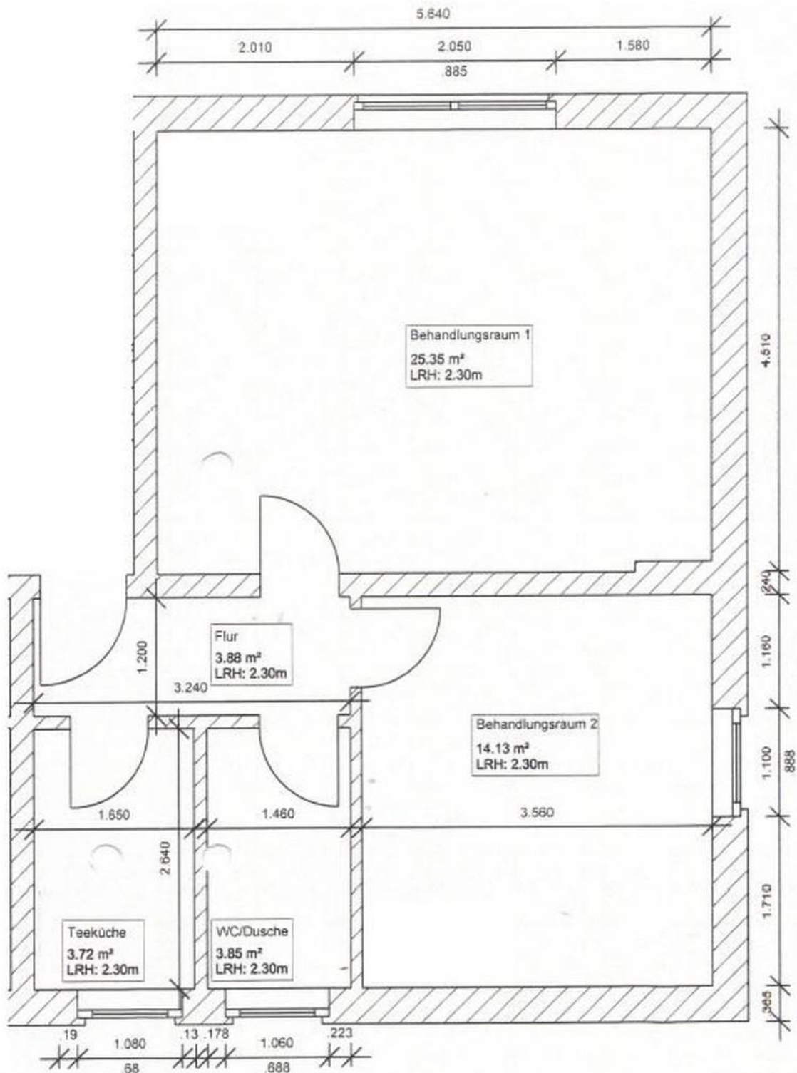
Grundriss
