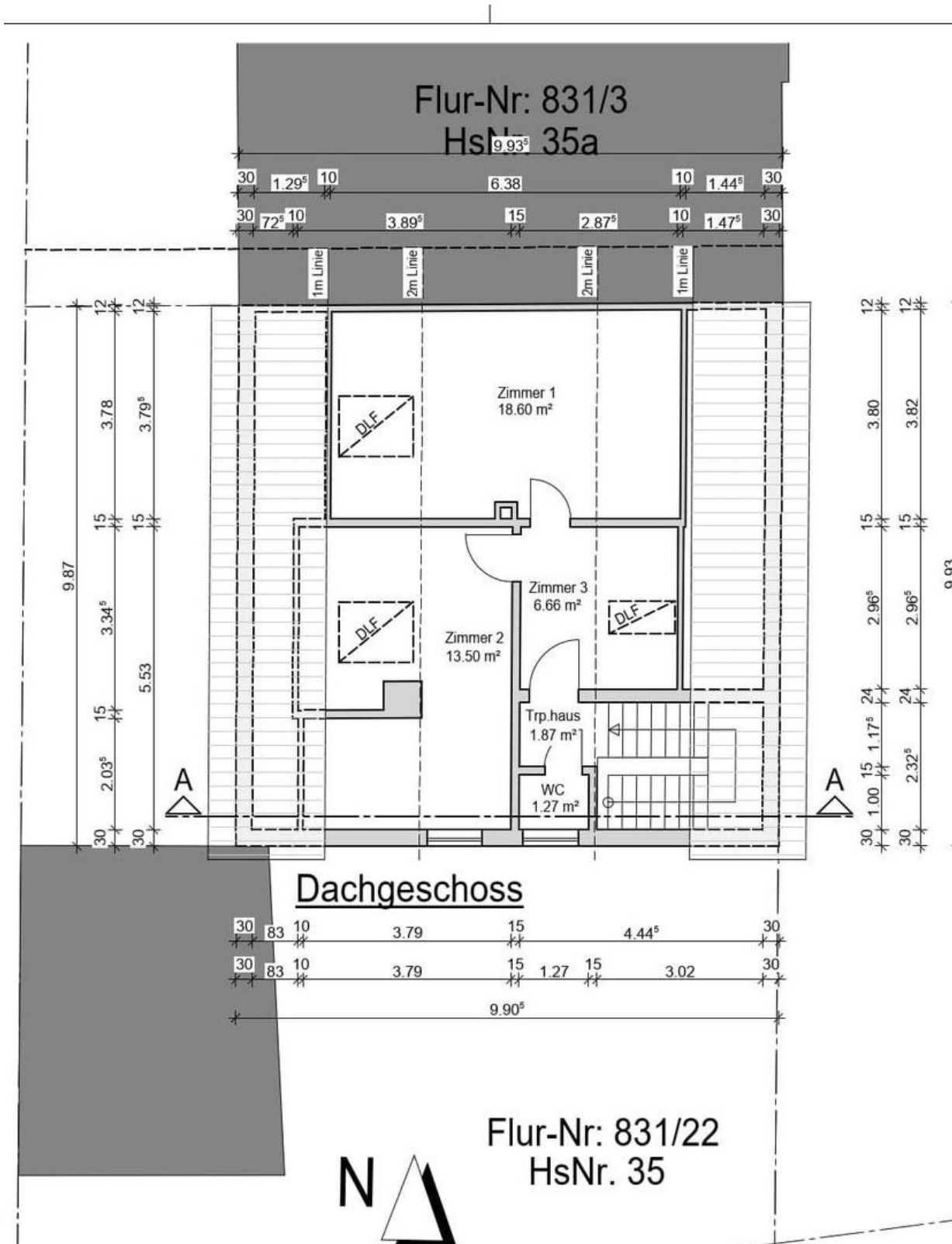
Grundrissplan DG
