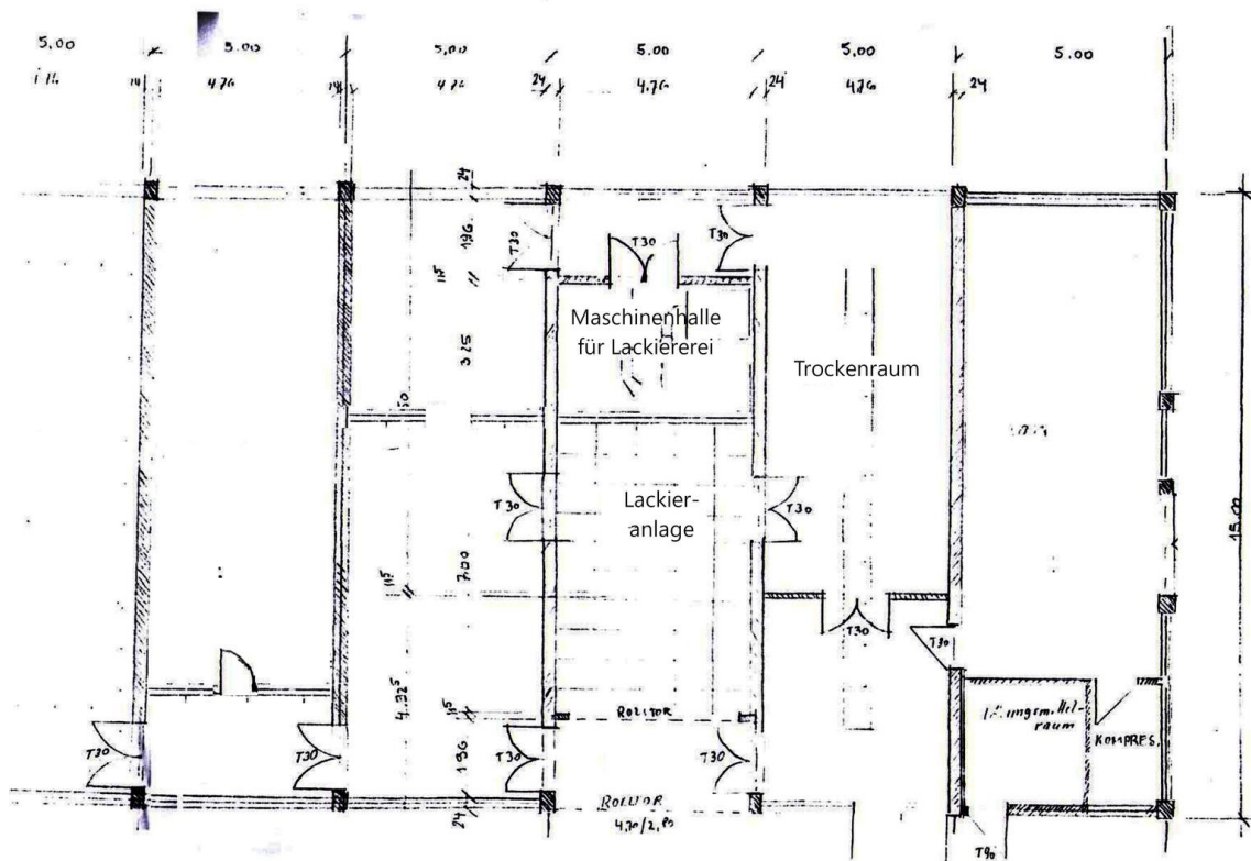
Grundriss Lagerhalle
