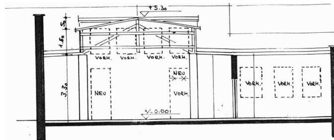
SCHNITT A-A
