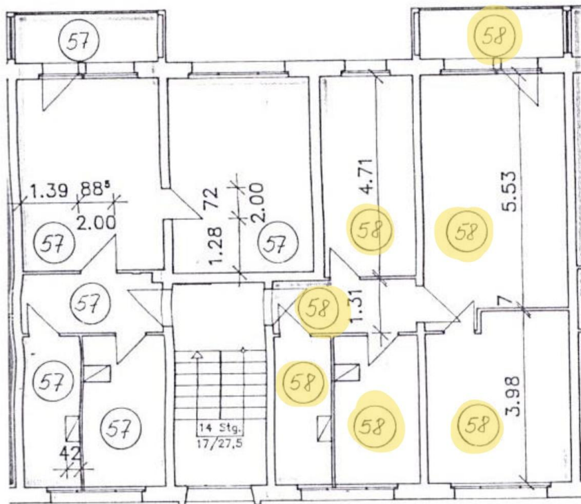
Grundriss
