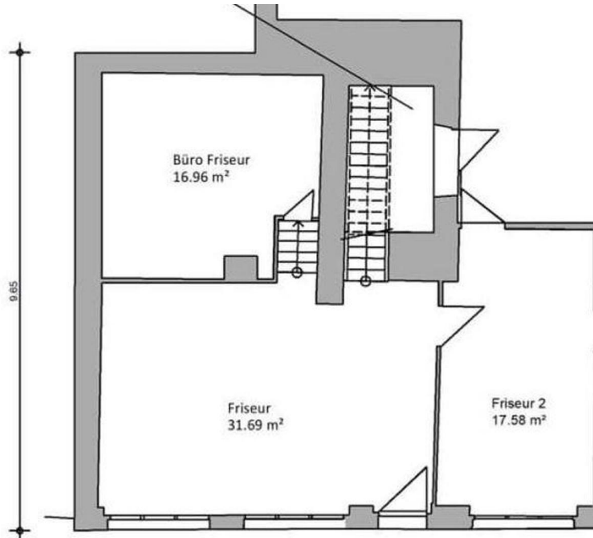
Grundriss EG Laden
