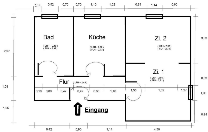
- Grundriss - Marktstrasse 149 / 3 1.OG
