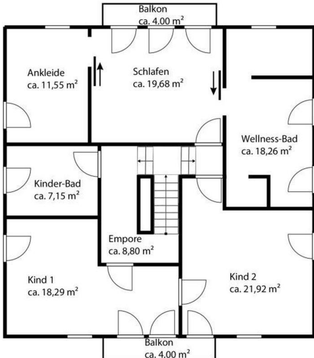
Grundriss OG
