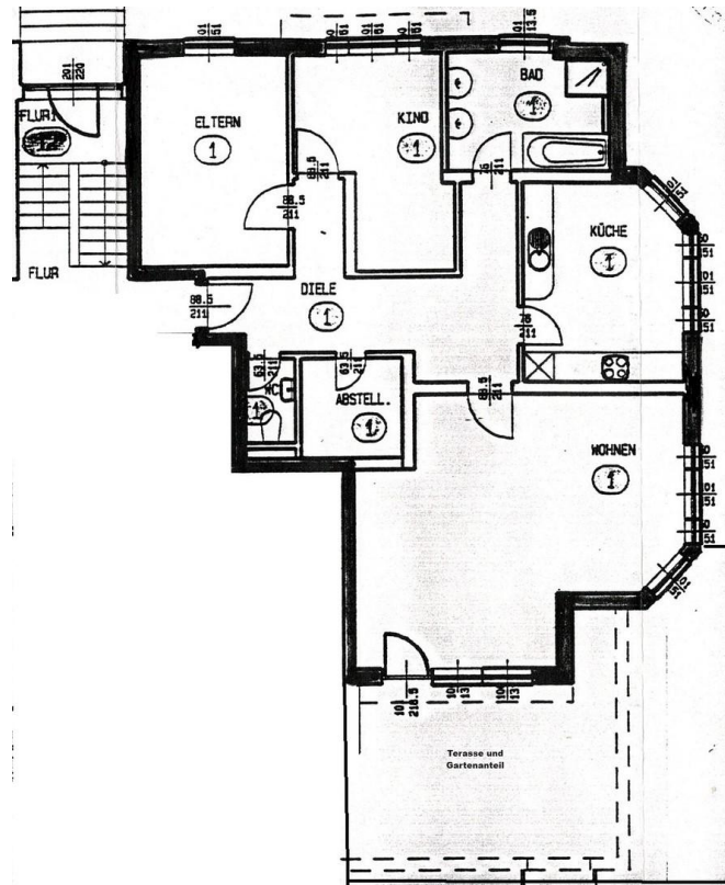
Grundriss
