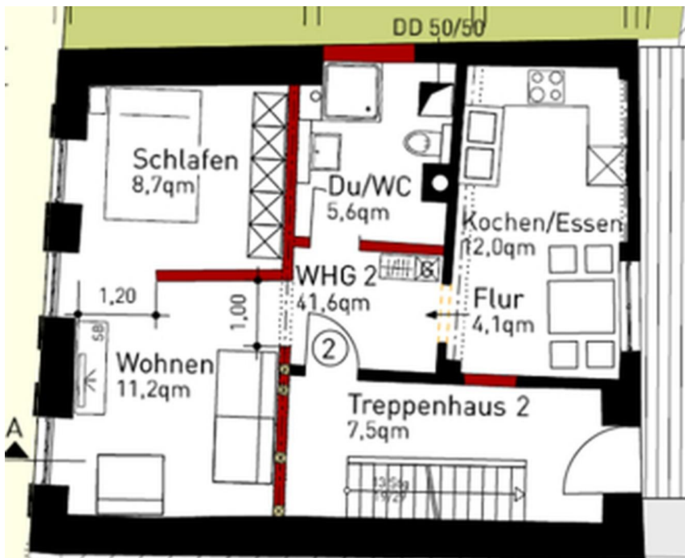
Wohnungsgrundriss
