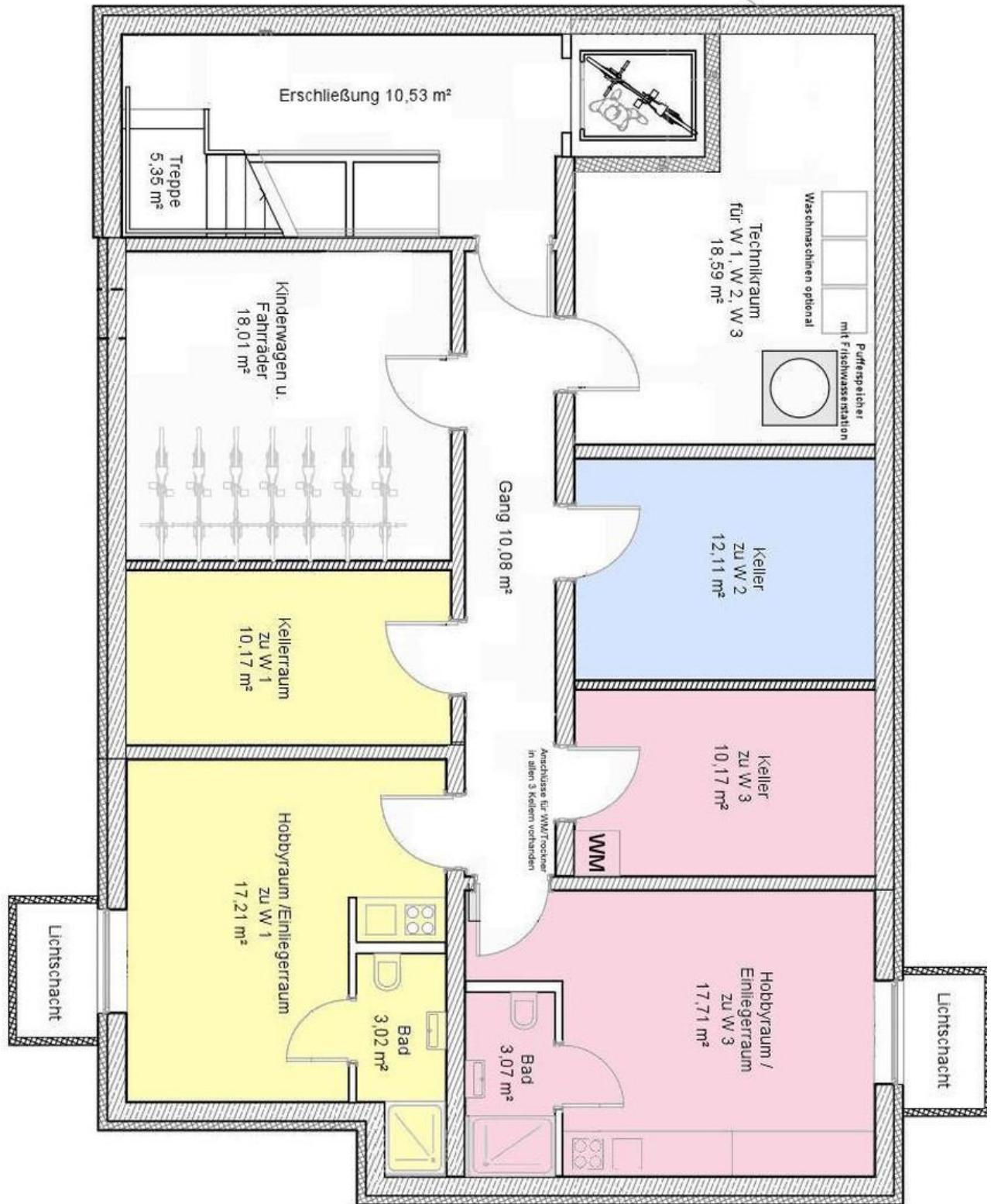
Grundriss Untergeschoß
