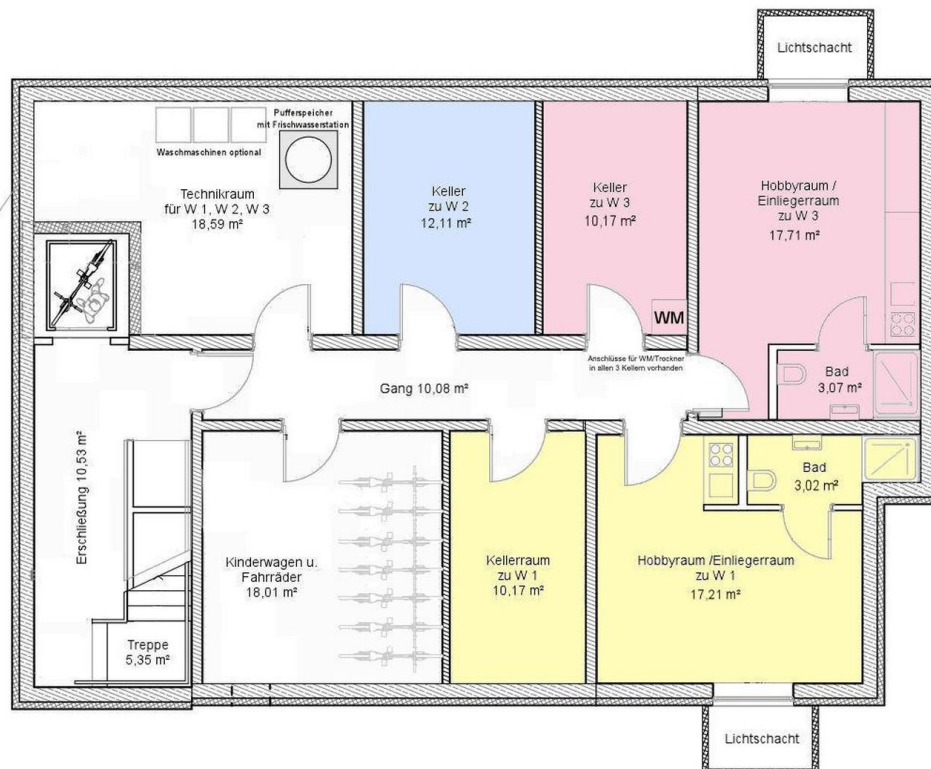
Grundriss Untergeschoß
