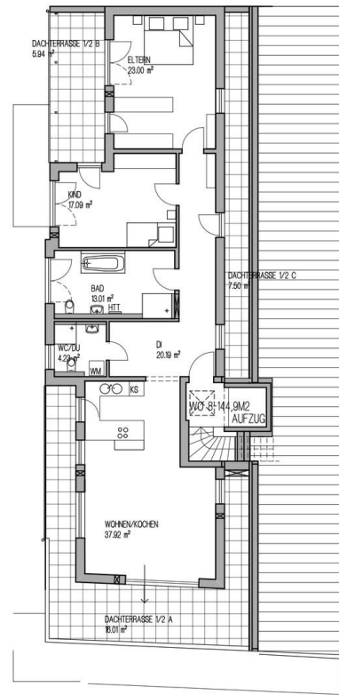
Grundriss
