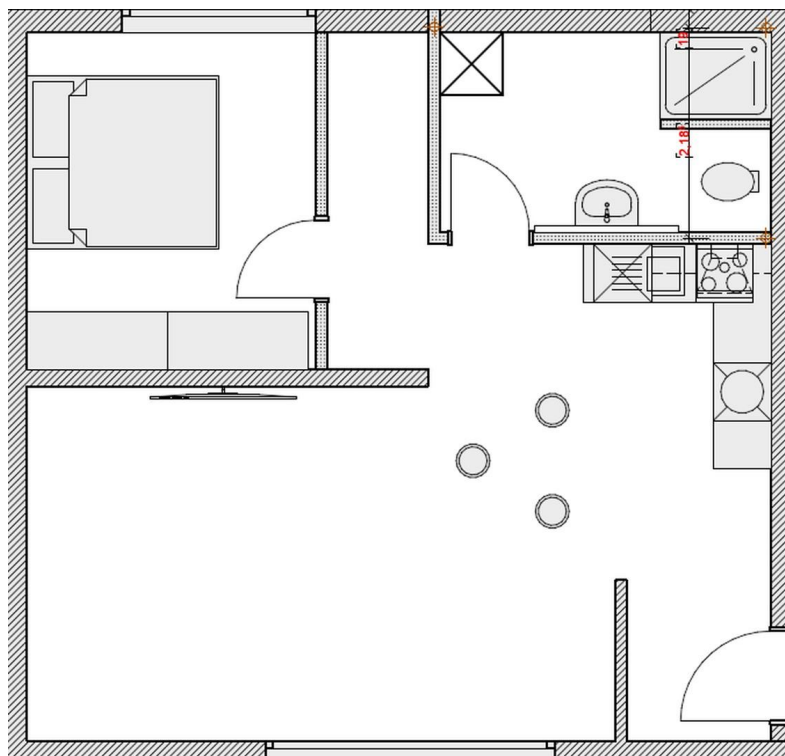
Grundriss
