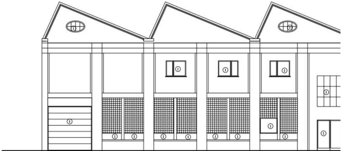
Ansicht - Vorderseite
