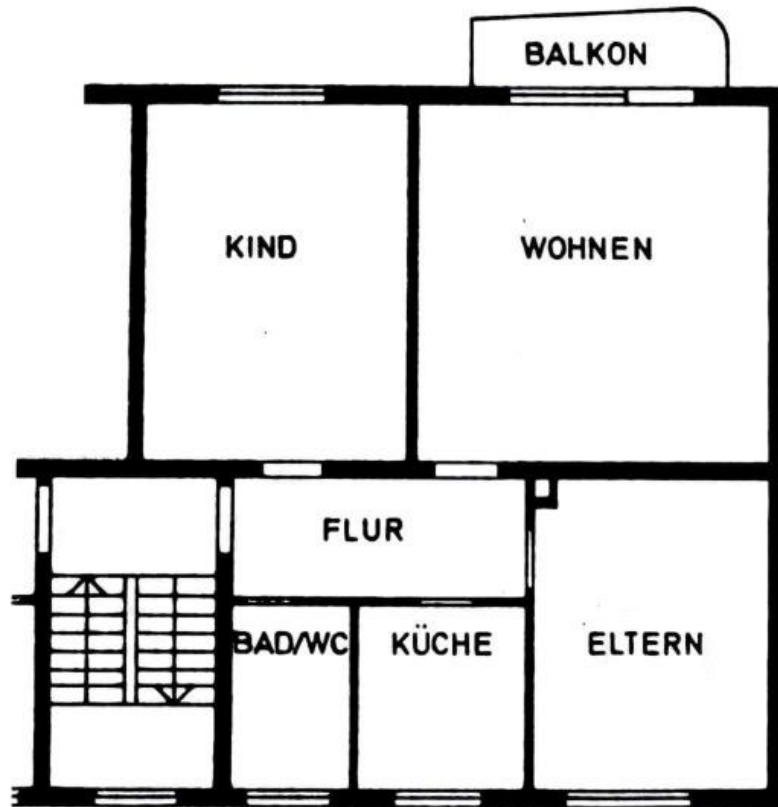
3 ZIMMERWOHNUNG M 1:100
