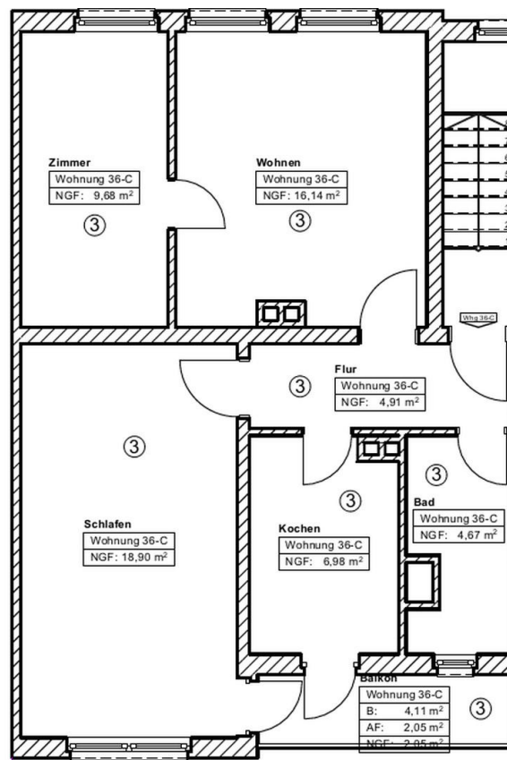
Grundriss
