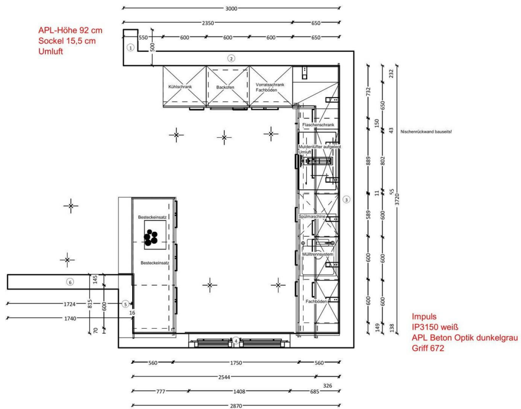
Plan neue Einbauküche
