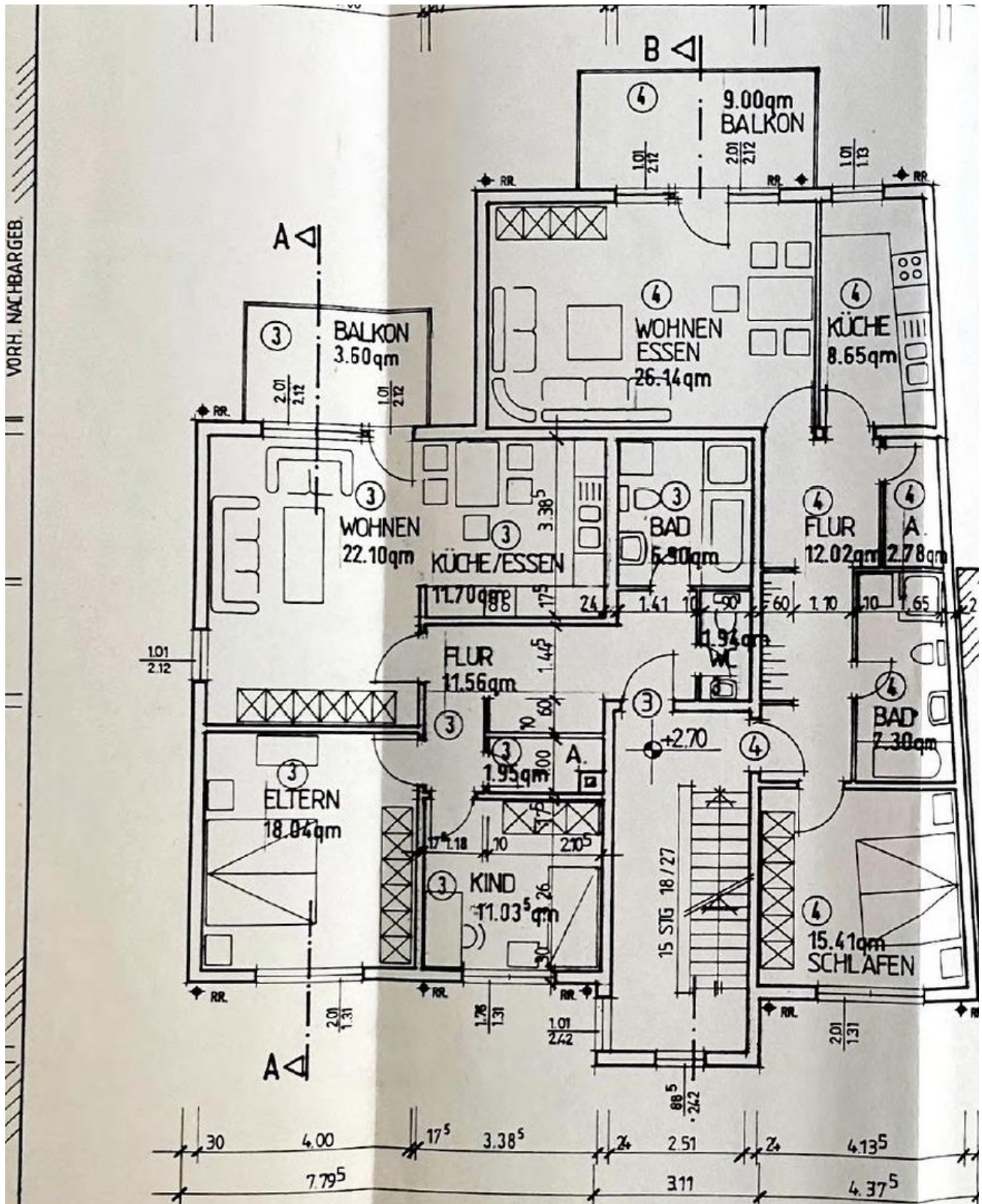
Grundriss Wohnung №4
