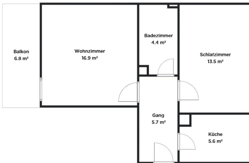
Grundriss 2-Zi Wohnung
