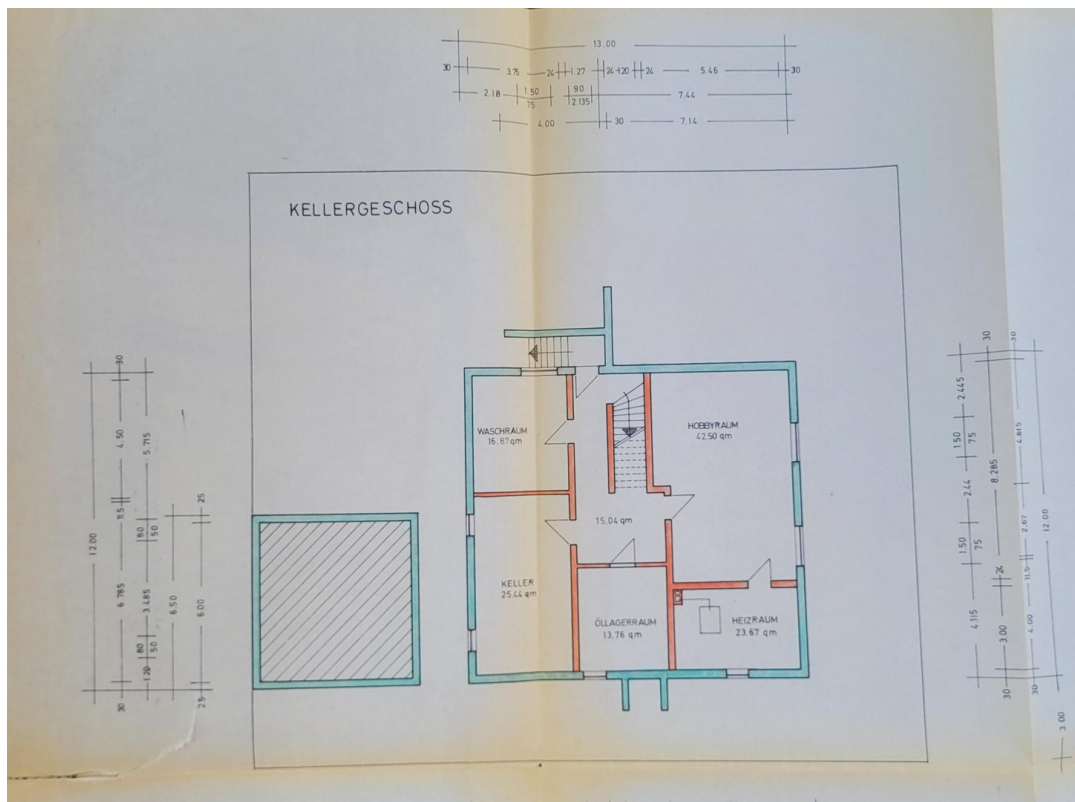
Grundriss KG
