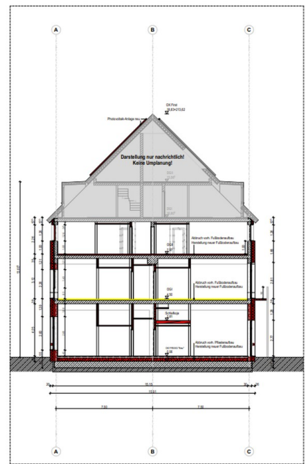
Querschnitt B
