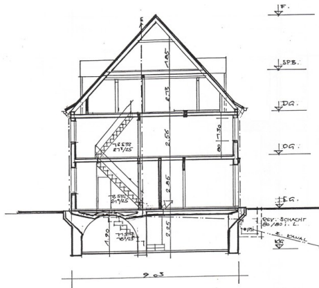
QUIRSCHNITT
