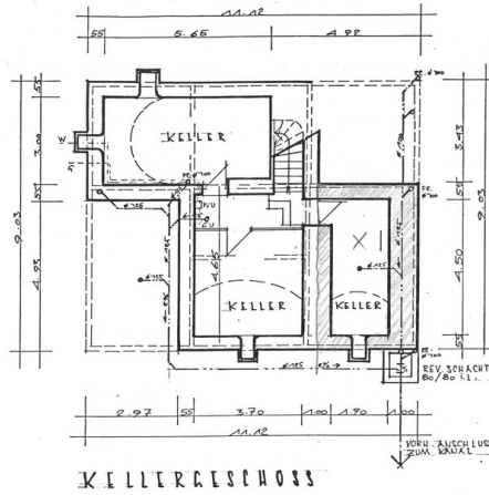
KELLERGESCHOSS
