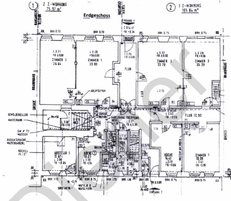
Grundriss Erdgeschoss
