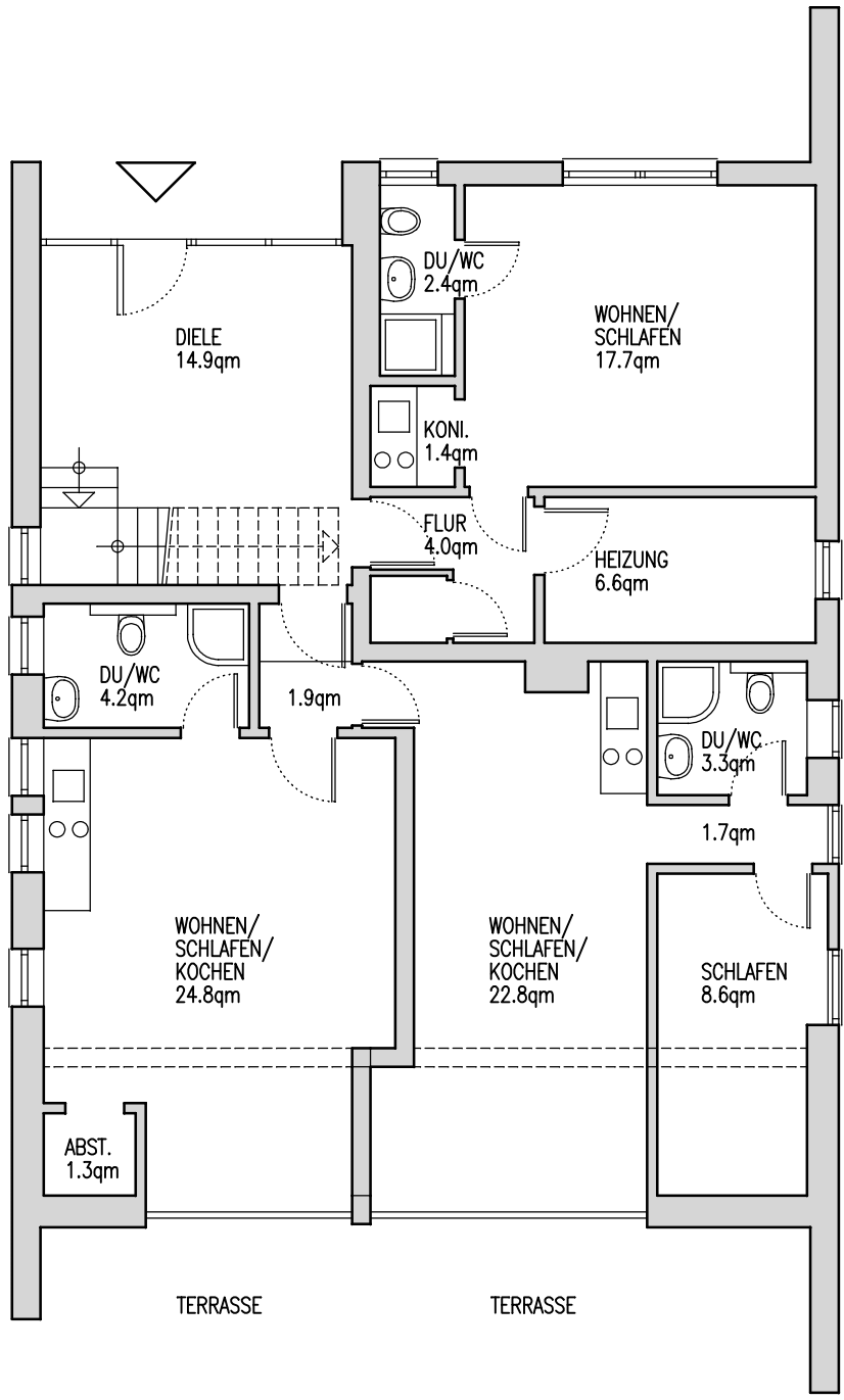
ERDGESCHOSS
