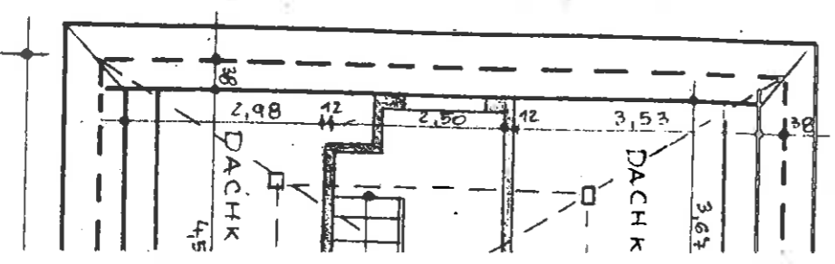
DACHGESCHOSS
