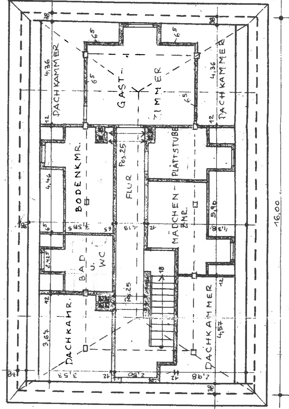
DACHGESCHÖß
