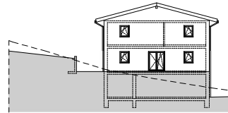
ANSICHT WEST
