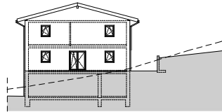
ANSICHT OST
