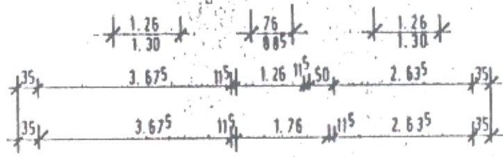
ERDGESCHOSS M. 1:100
