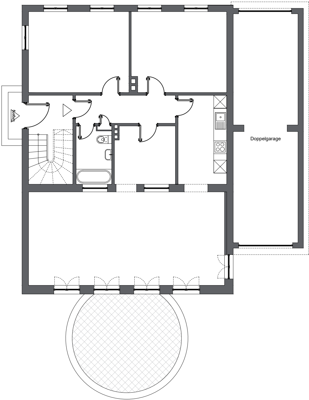
EG Grundriss
