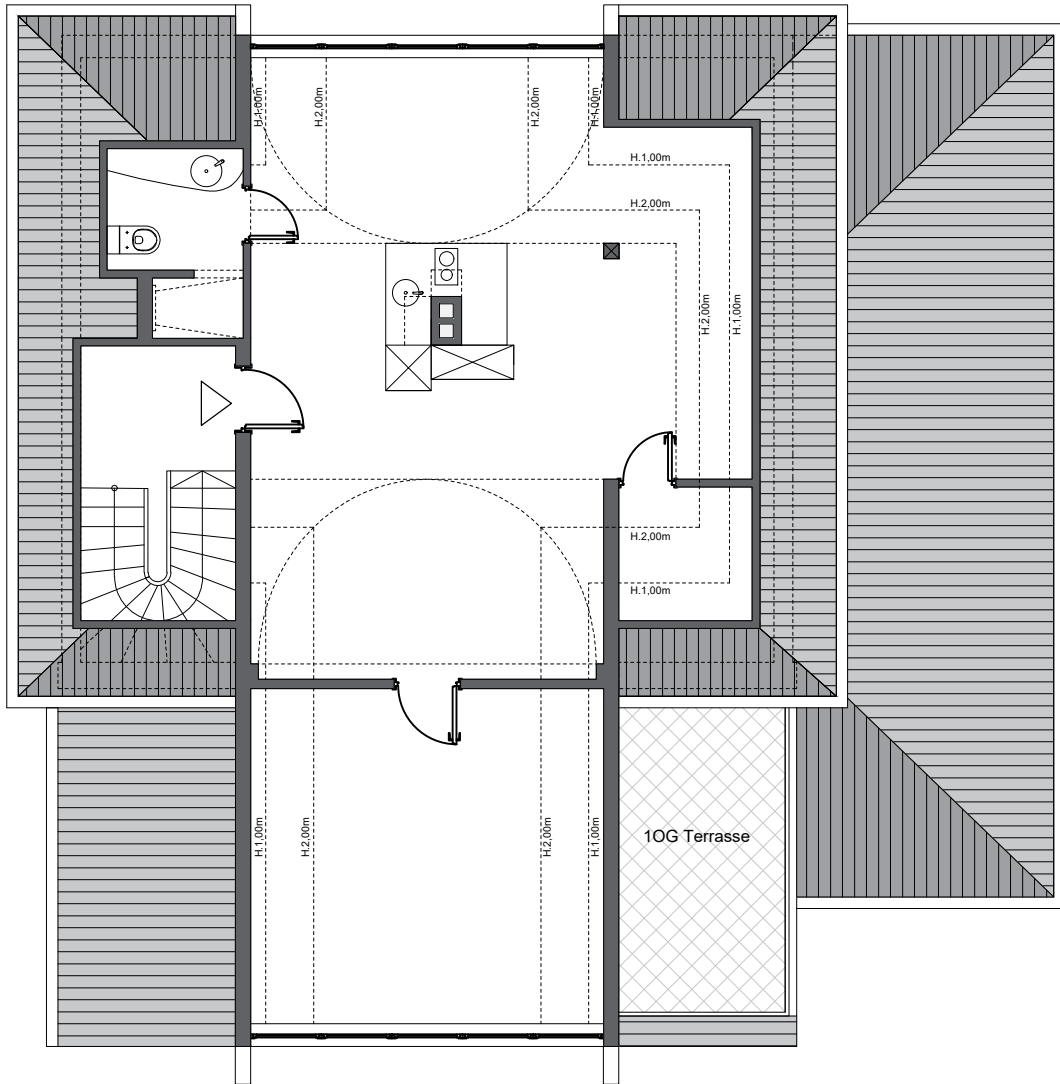
DG Grundriss
