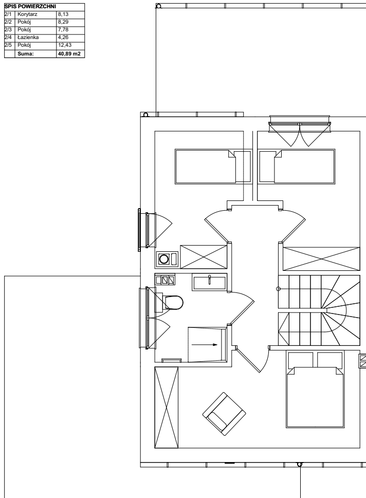
PODDASZE RZUT
