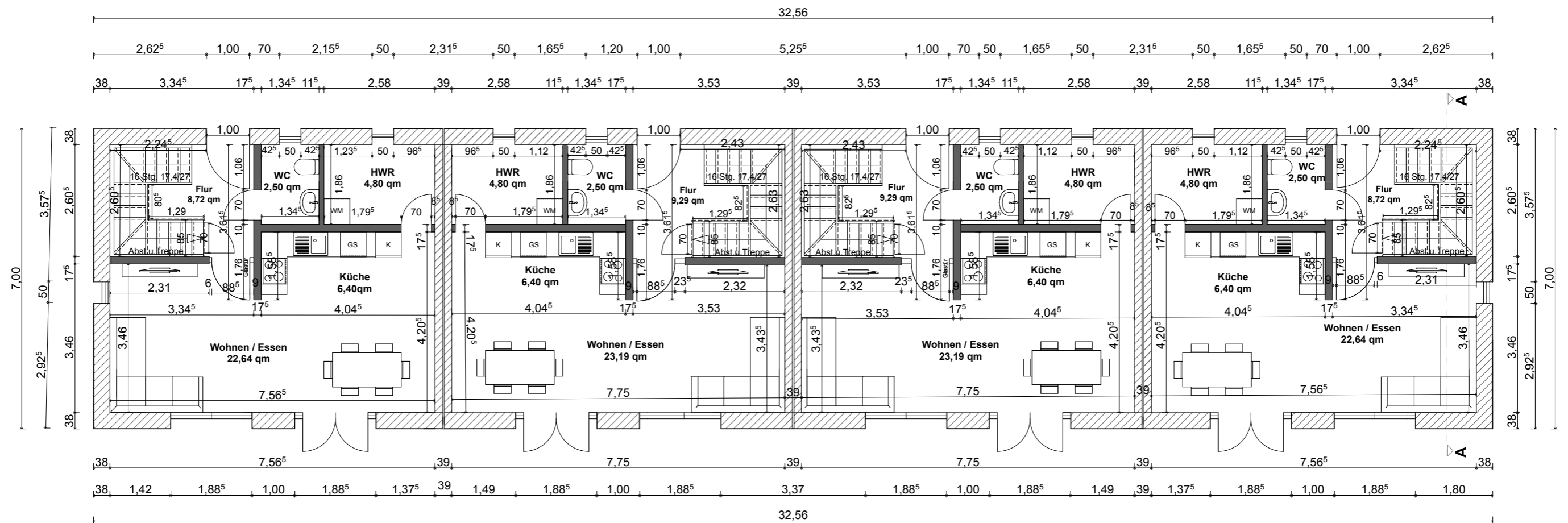
Erdgeschoss
