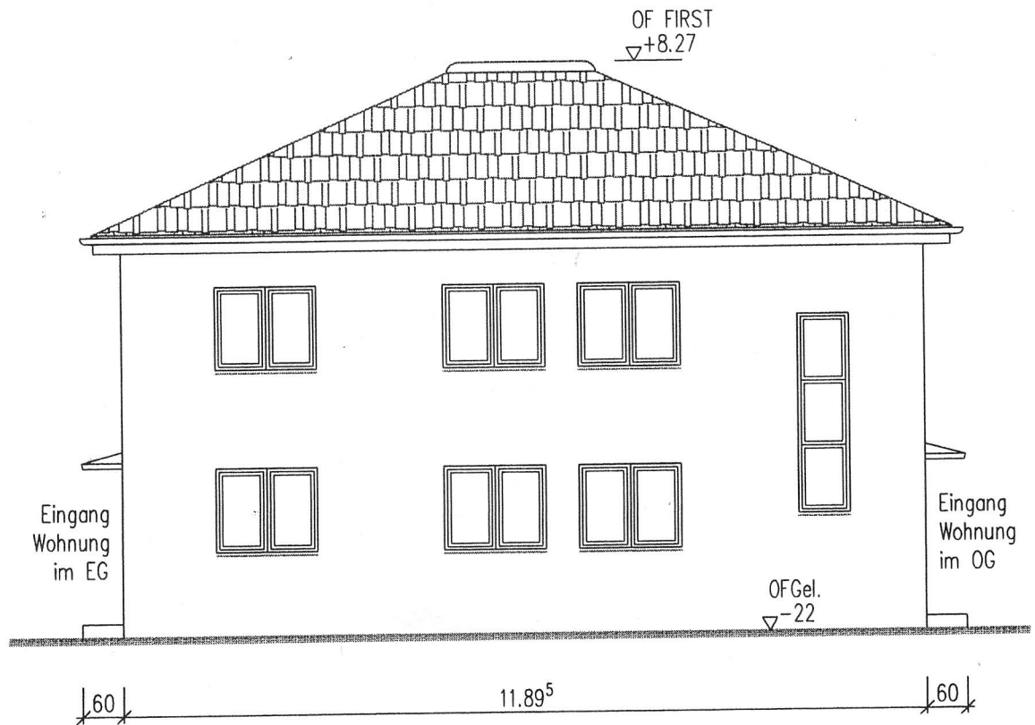
Ansicht von Westen Straßenfassade
