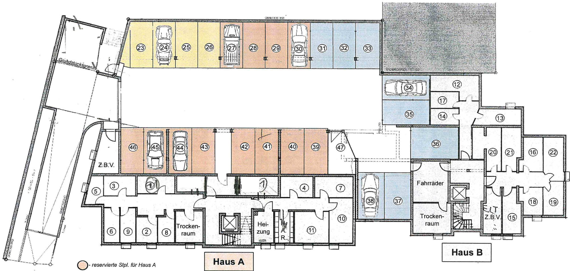
- Keller- und Tiefgaragenplan -
