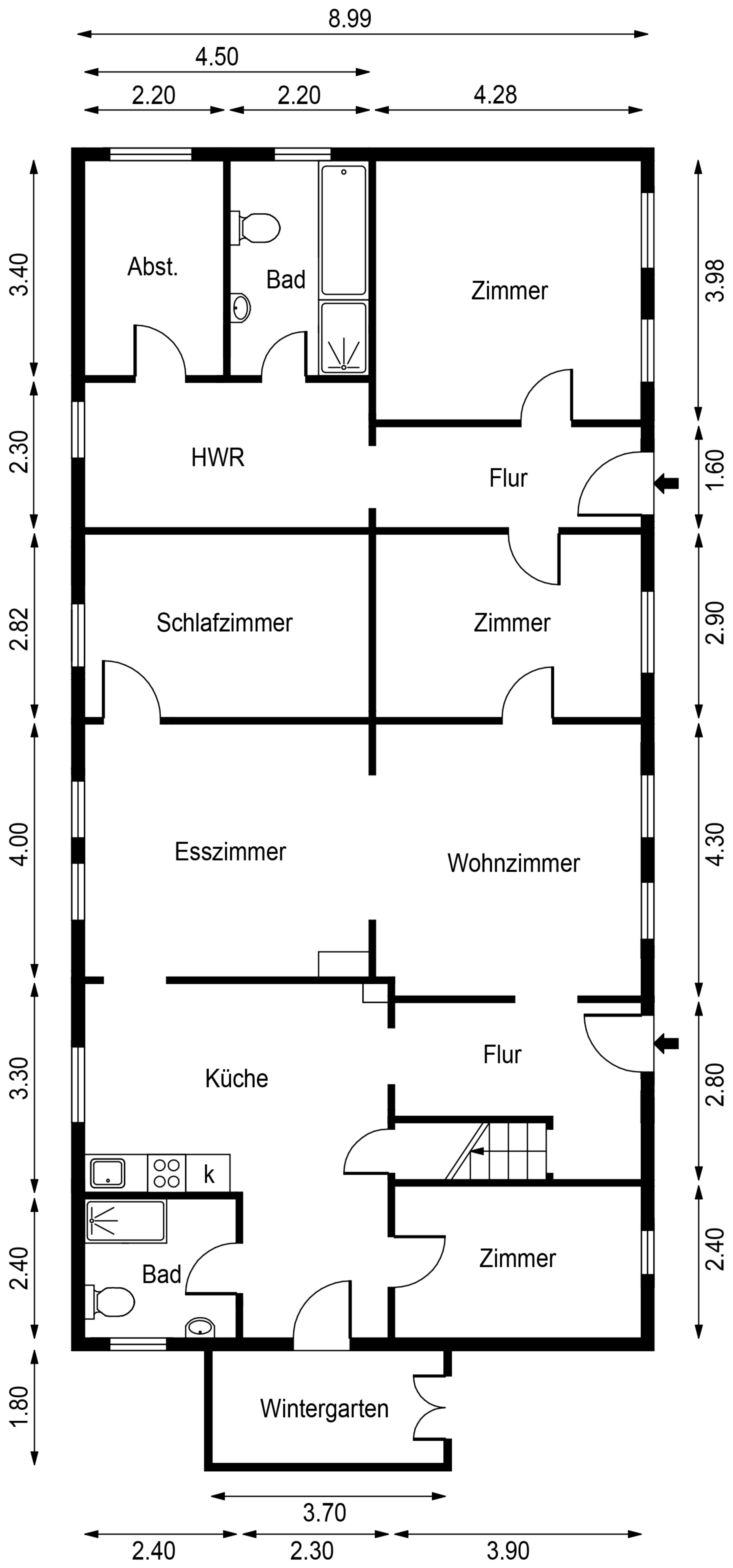
Erdgeschoss
