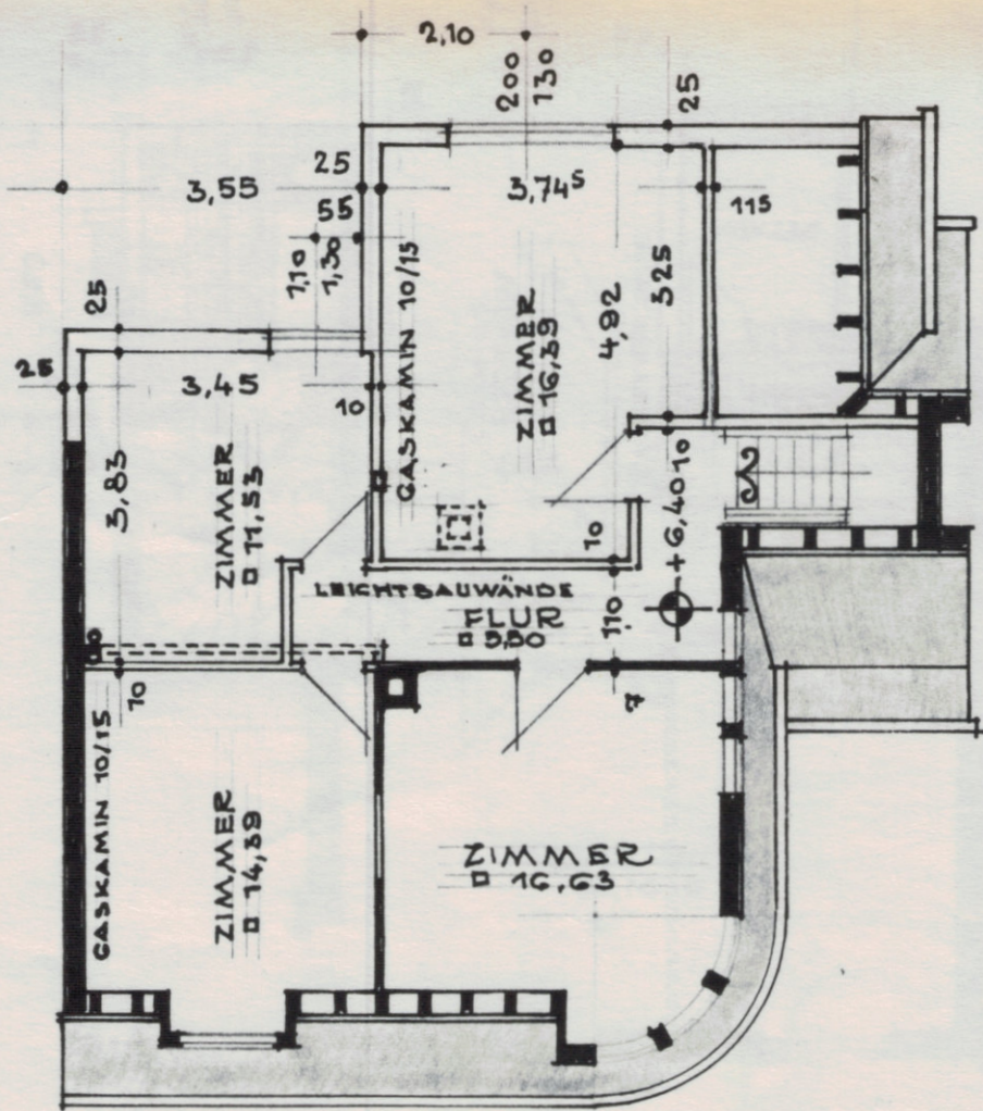
DACHGESCHOSS
