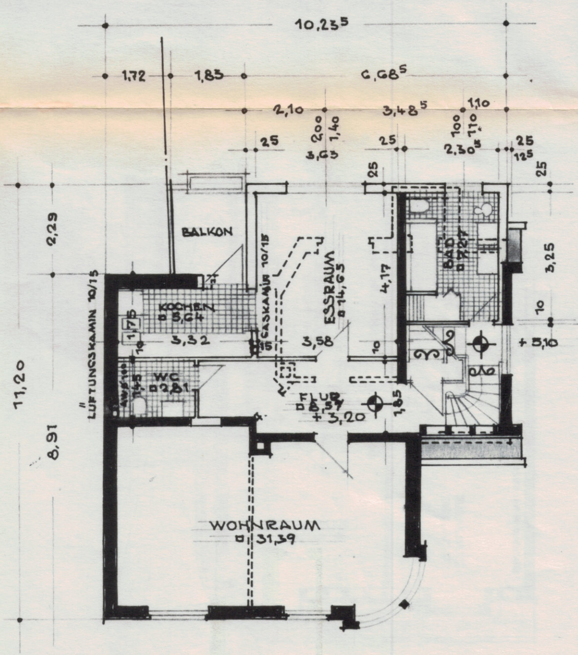
1. OBERGESCHOSS
