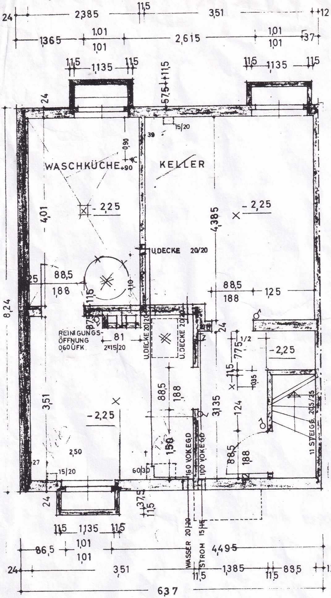
KELLERGESCHOSS
