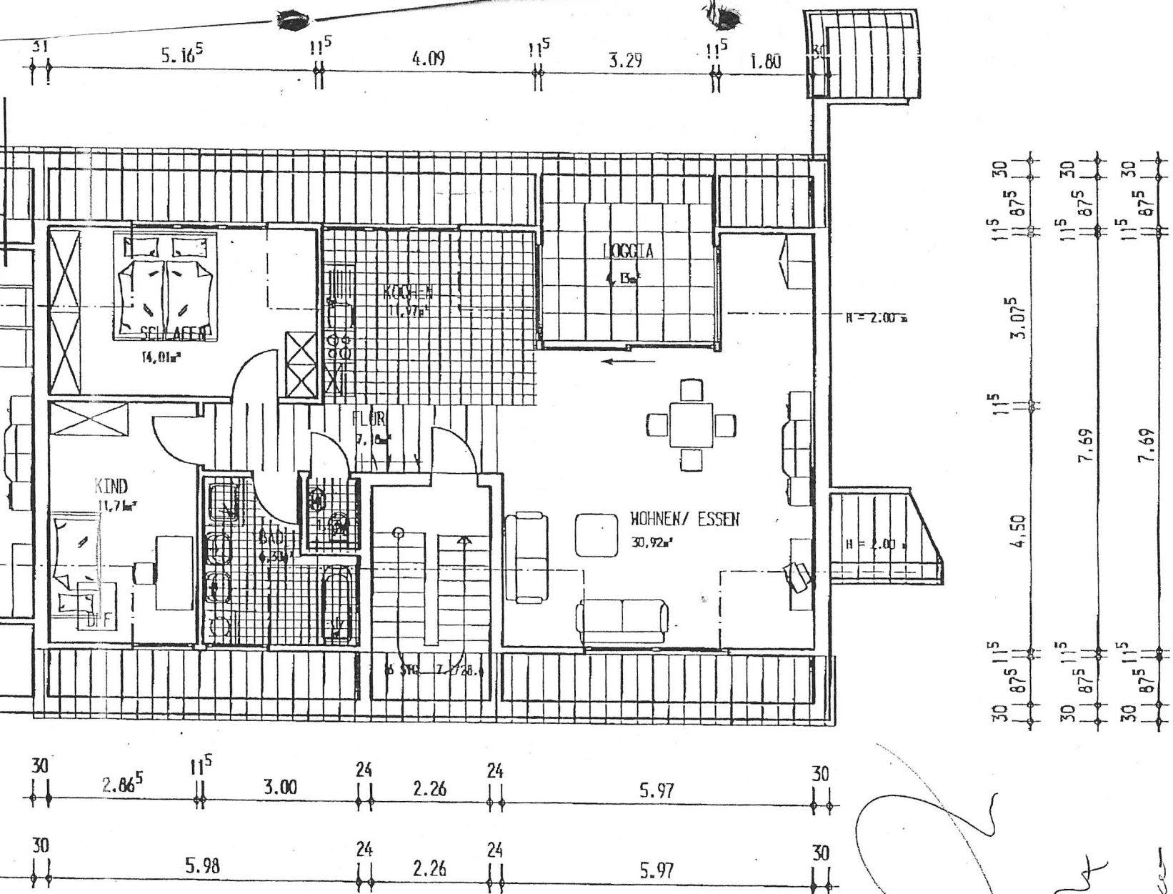
Werkplan Dachgeschoss
