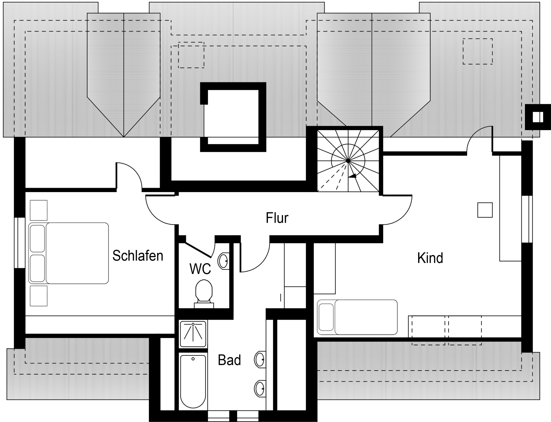
2. Dachgeschoss
