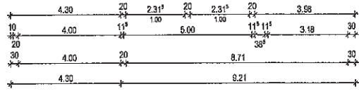
Grundriss Dachgeschoss
