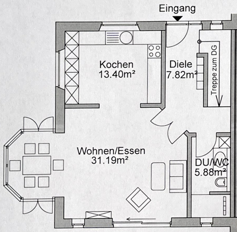
Grundriss Erdgeschoss Westerhörn 4, Wenningstedt (Whg. 2)
