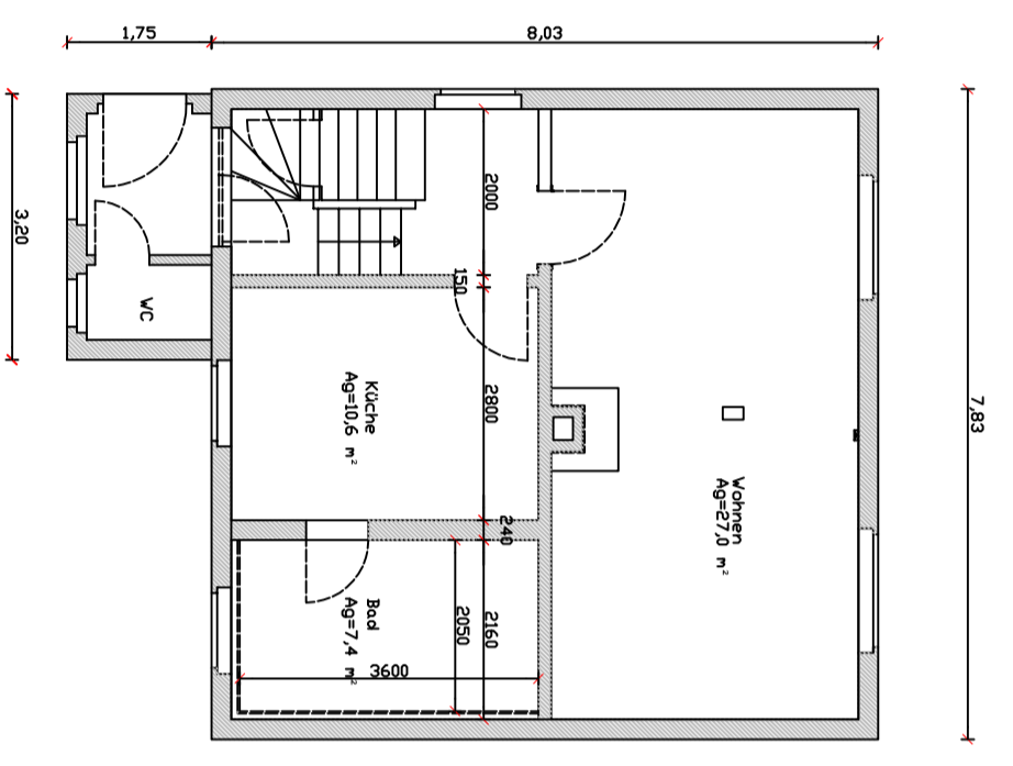
Grundriß EG
