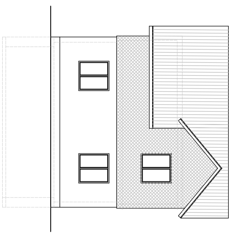
Ansicht- SO
