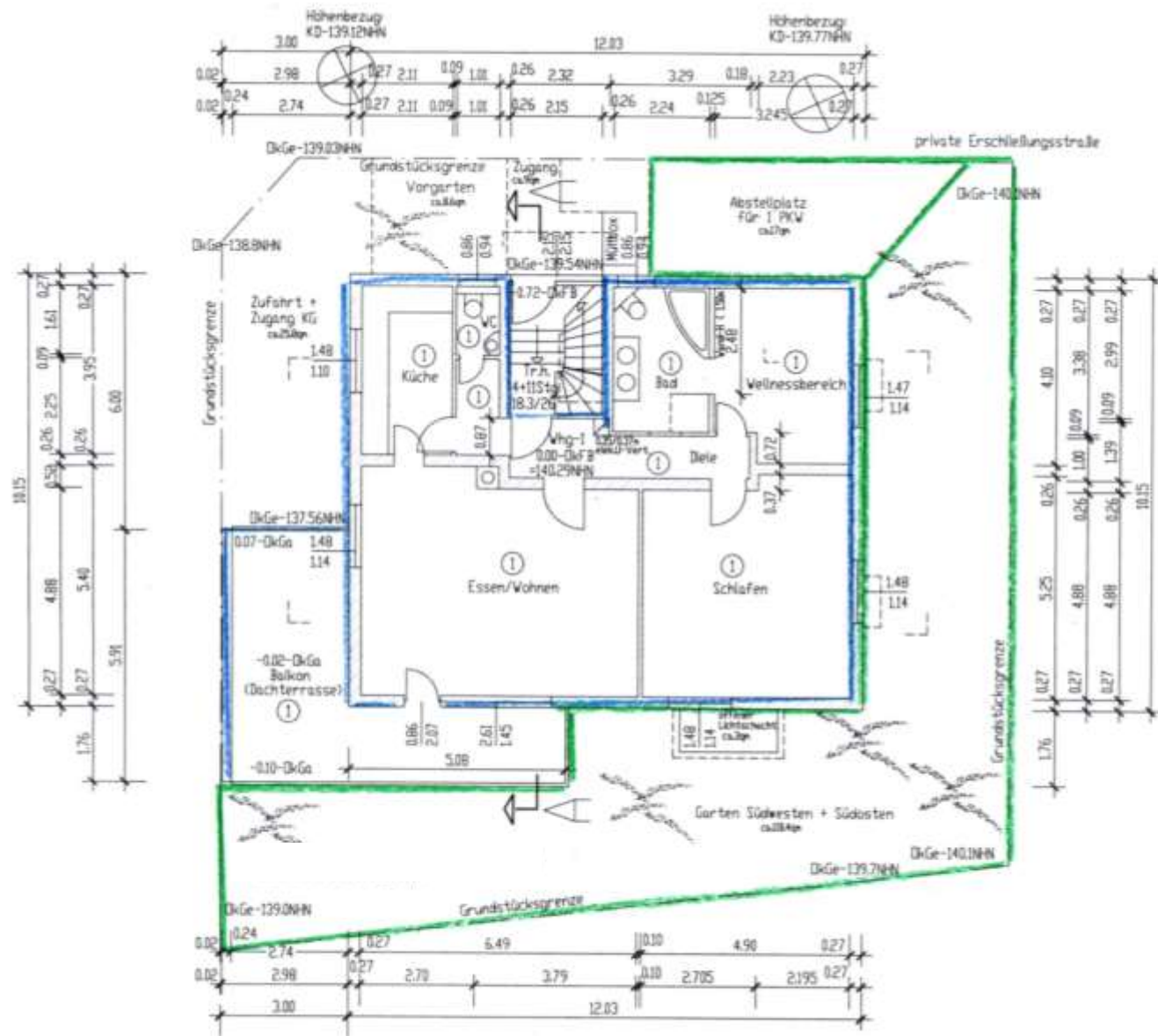
Erdgeschoss + Freiflächen
