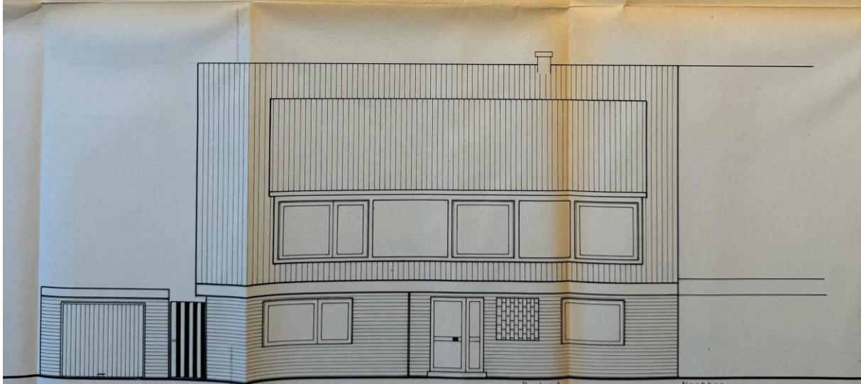
RÜCKANSICHT
