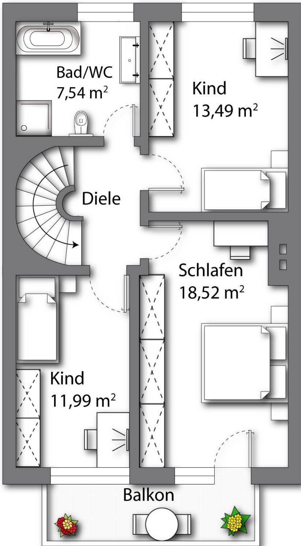
Obergeschoss
