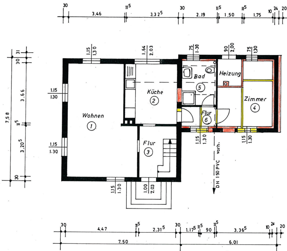
Erdgeschoß
