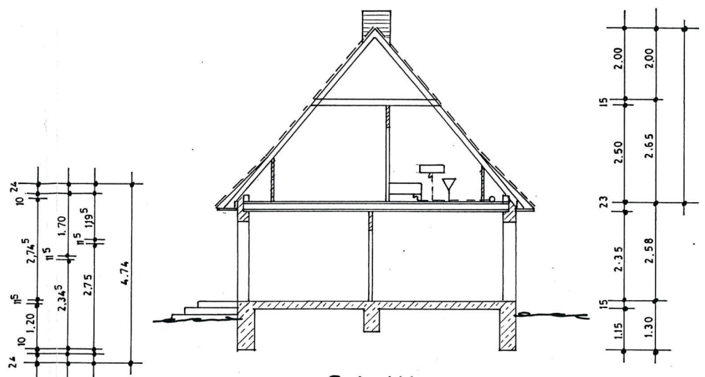
Schnitt
