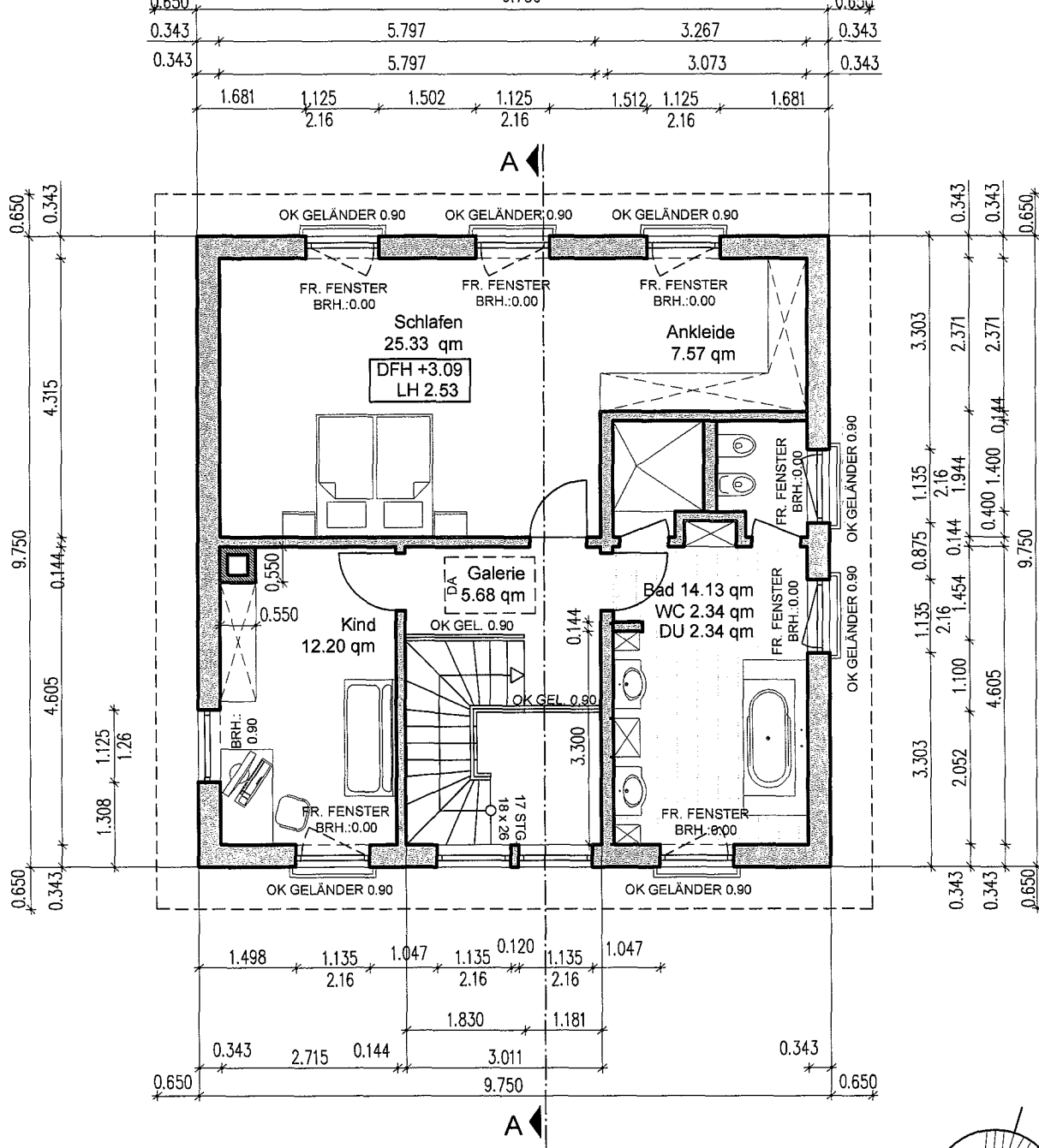
Dachgeschoß
