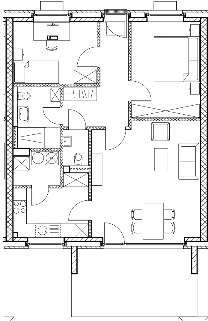
ERDGESCHOSS WOHNUNG 01 LINKS
