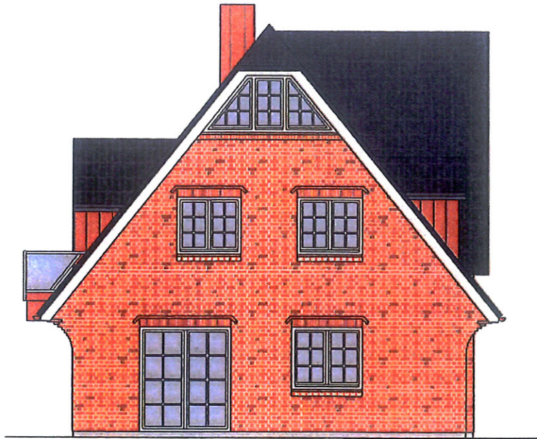
Ostansicht
